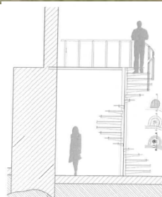
Planos de detalle de la nueva escalera
