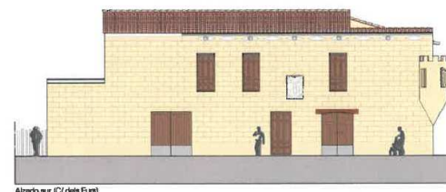
Alzado sur (C/ de la Fara)
