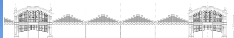
ALZADO SUROESTE
