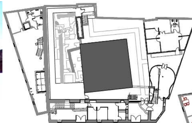
ESTAT ACTUAL PLANTA BAIXA AJUNTAMENT
